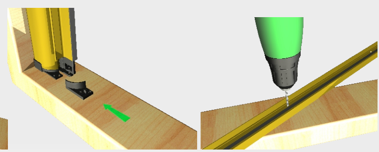
Praticare n.3 fori al profilo di chiusura
