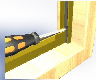
Inserire il cassonetto prima nel supporto chiuso poi farlo aderire al vano inserendolo nel supporto aperto e inserire il tappo di chiusura
