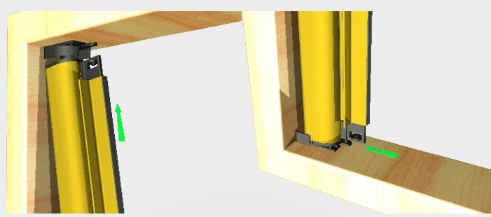
Inserire il cassonetto prima nel supporto chiuso poi farlo aderire al vano inserendolo nel supporto aperto e inserire il tappo di chiusura
