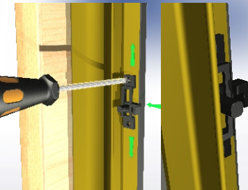
Fissare l'aggancio si sicurezza
