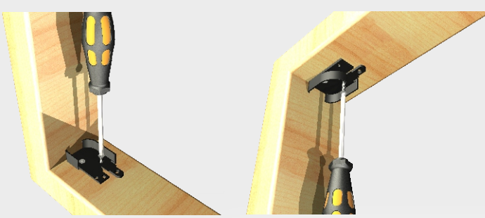
Fissare i supporti nel vano sup. + inf.
