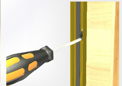
Regolare l'aggancio e fissarlo
