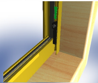
Inserire il cassonetto prima nel supporto chiuso poi farlo aderire al vano inserendolo nel supporto aperto e inserire il tappo di chiusura
