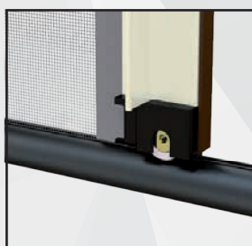
Particolare scivolo a ruota.
