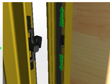
Fissare il gancio di sicurezza poi regolare il gancio presente nel profilo di chiusura in modo che possa agganciare e bloccarlo
