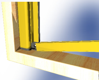
Inserire le guide tra il cassonetto e il profilo di chiusura e portarlo a contatto con il vano e bloccare tramite i fermi
