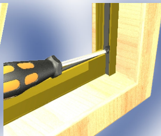
Inserire le guide tra il cassonetto e il profilo di chiusura e portarlo a contatto con il vano e bloccare tramite i fermi
